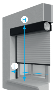
Enroulement extérieur Implantation N°2 : coulisse MA Implantation N°3 : coulisse MS
