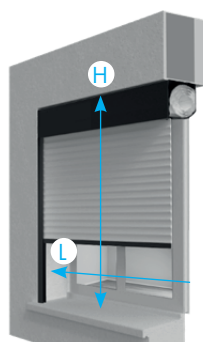
Enroulement intérieur Implantation N°1 : coulisse MA et caisson 2x20°
